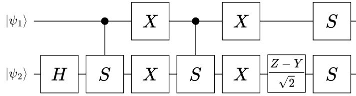
Рис. 2: Алгоритм квантового вентиля CNOT, реализованного с помощью CZ вентиля с динамической отвязкой от окружения
